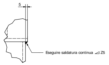
Det. "A" Scala (1 : 2)
